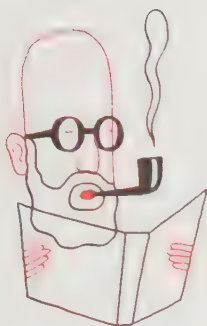
WISE
