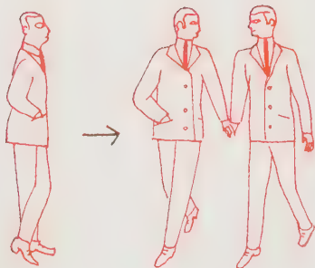
MAN
