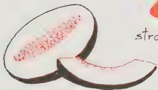
melon
